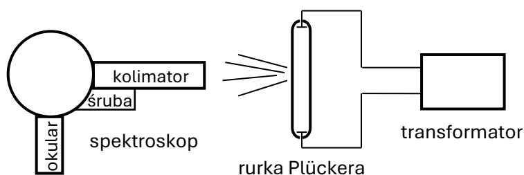
Rys. 10. Schemat układu pomiarowego
