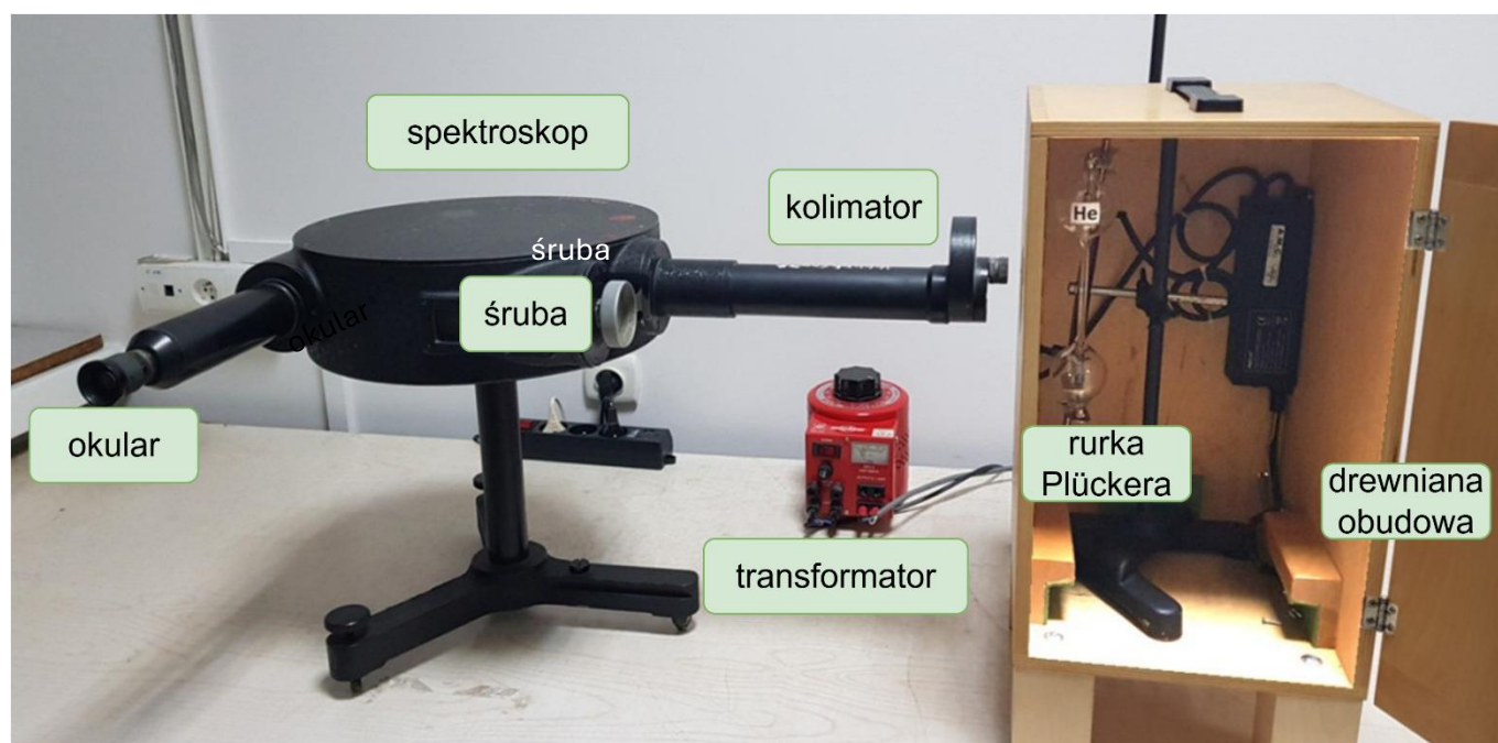
Rys. 11. Rzeczywisty wygląd stanowiska pomiarowego
