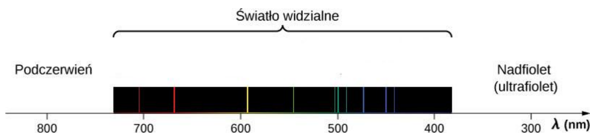
Rys. 3. Widmo emisyjne w świetle widzialnym dla helu
