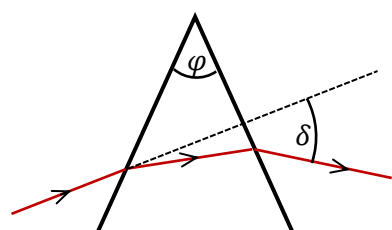
Rys. 6. Załamanie światła w pryzmacie.
