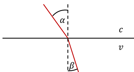
Rys. 5. Bieg światła w pobliżu powierzchni rozgraniczającej dwa ośrodki.
