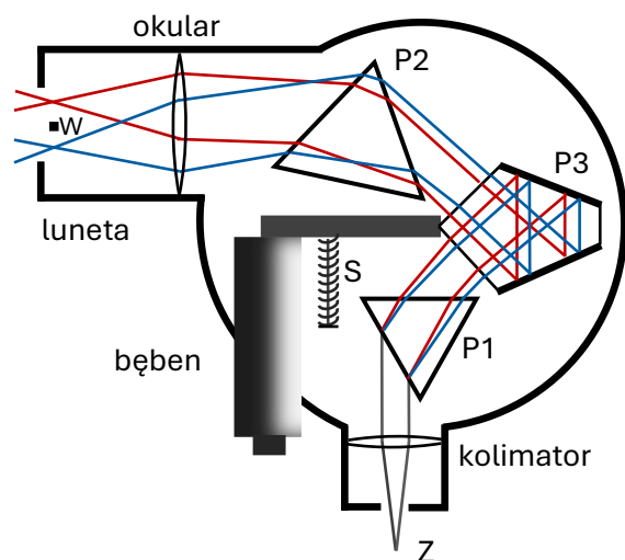
Rys. 9. Spektrometr pryzmatyczny
