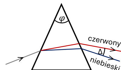
Rys. 7. Dyspersja światła w pryzmacie
