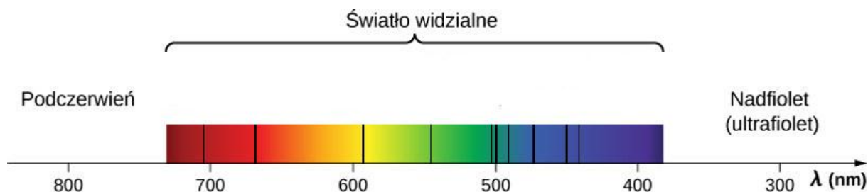
Rys. 4. Widmo absorpcyjne w świetle widzialnym dla helu
