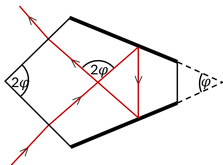
Rys. 8. Pryzmat pięciokątny
