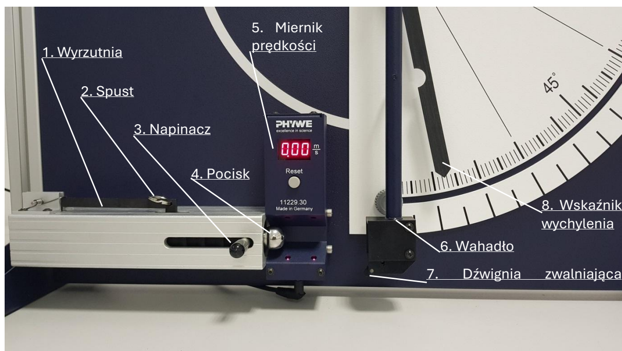
Rys. 3. Urządzenie pomiarowe
